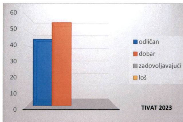
Figura 5 - Prikaz mikrobiološkog kvaliteta morske vode na javnim kupalištima u opštini Tivat tokom sezone 2023.g
