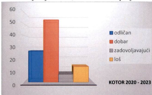
Figura 14 – Prikaz klasifikacije voda za kupanje za prethodne četiri sezone kupanja (2020. – 2023.g) u opštini Kotor
